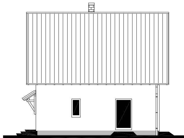
POHLED ZADNÍ
