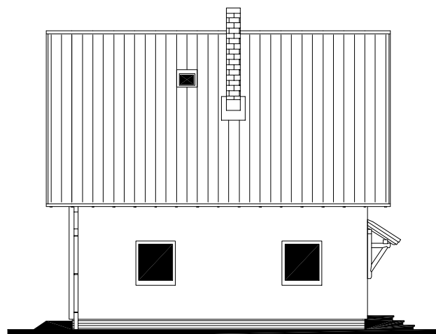
POHLED PŘEDNÍ
